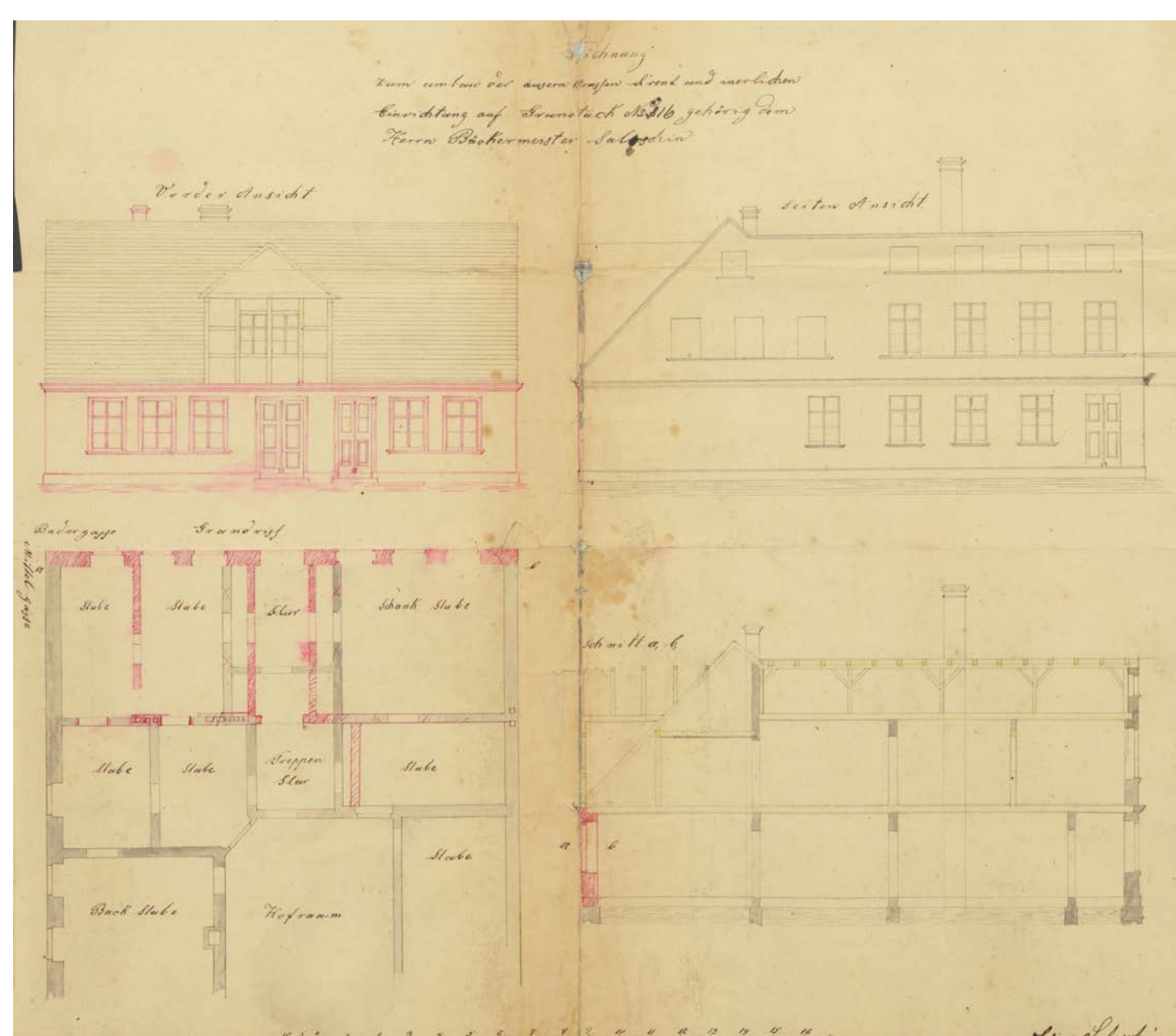
Eduard Wöhner, Projekt domu i piekarni macy Eliasa Saloschina (ulica Łaziebna 2), 1880 rok; zbiory: APL, Akta miasta Leszno, sygn. 2246, s. 3
