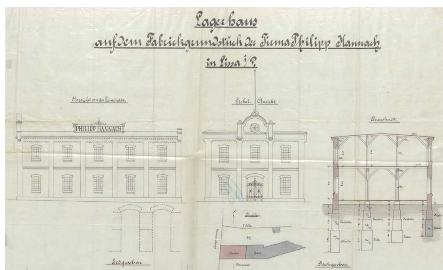
Heinrich Wittig, Projekt magazynu fabryki pomp, 1895 rok; zbiory: APL, Akta miasta Leszno, sygn. 2341, s. 103
