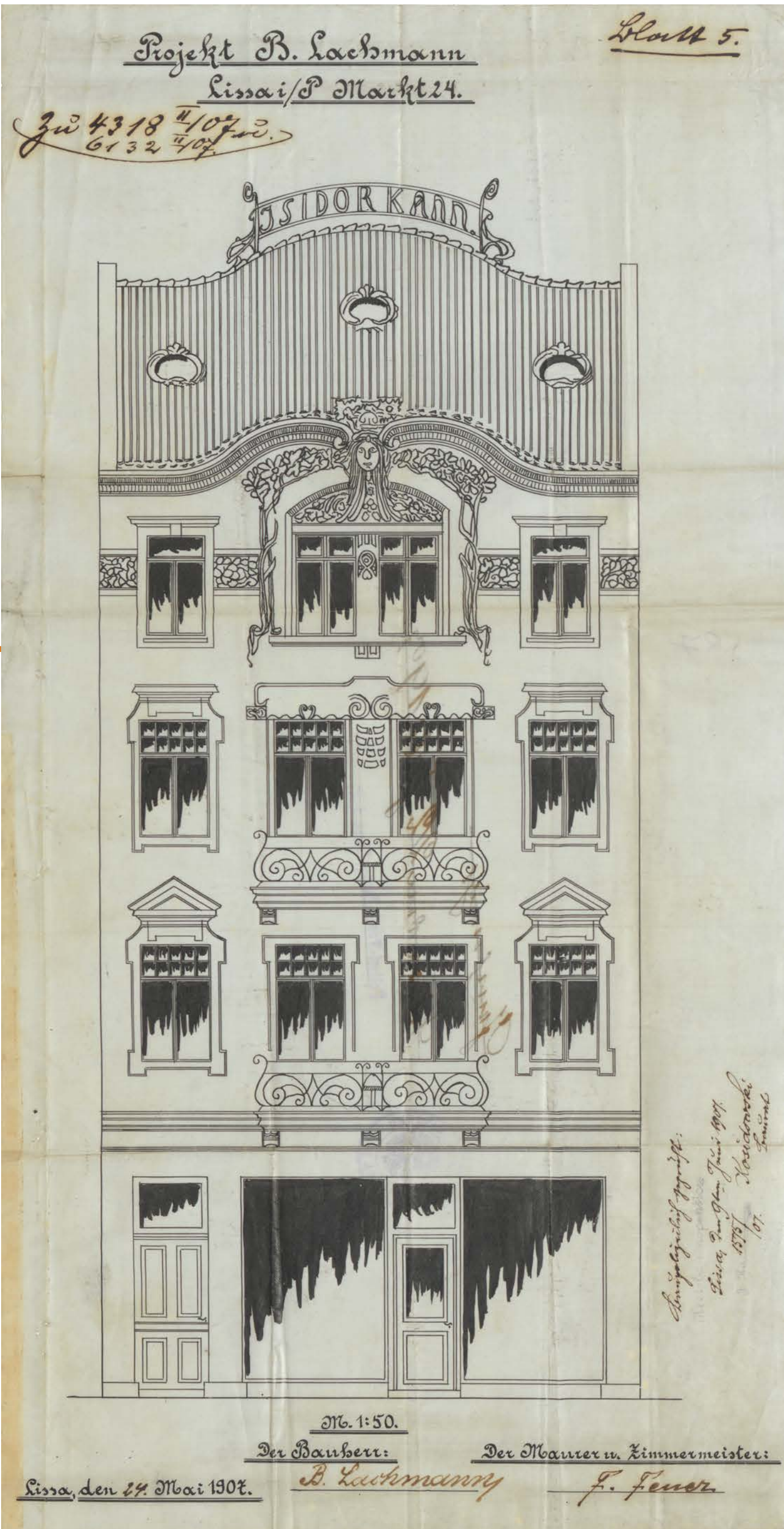
Franz Wittig, Projekt kamienicy rodziny Kannów (Rynek 24), 1907 rok; zbiory: APL, Akta miasta Leszno, sygn. 2533, s. 27
