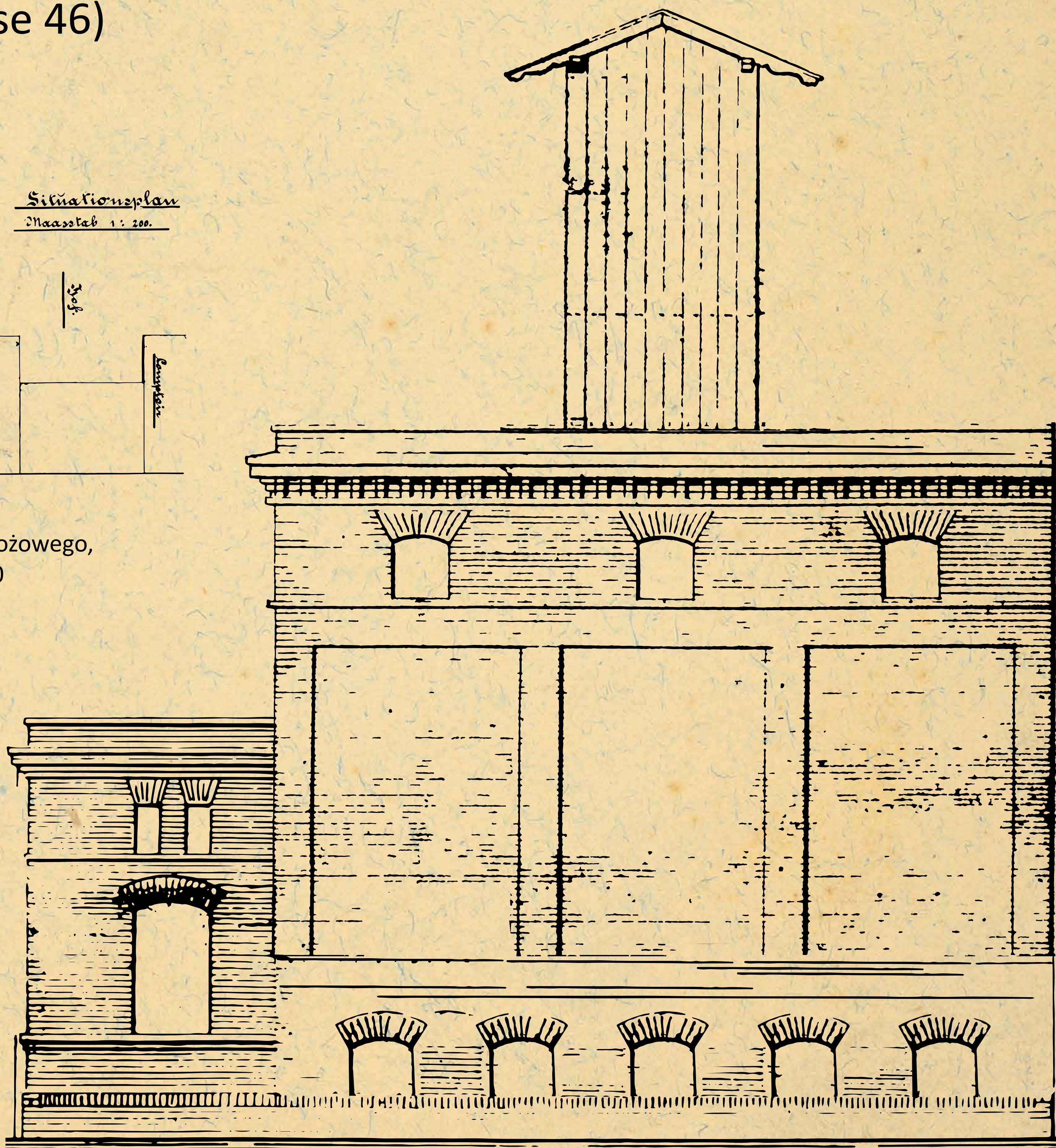
Fasada magazynu zbożowego, 1889, APL sygn. 2590
