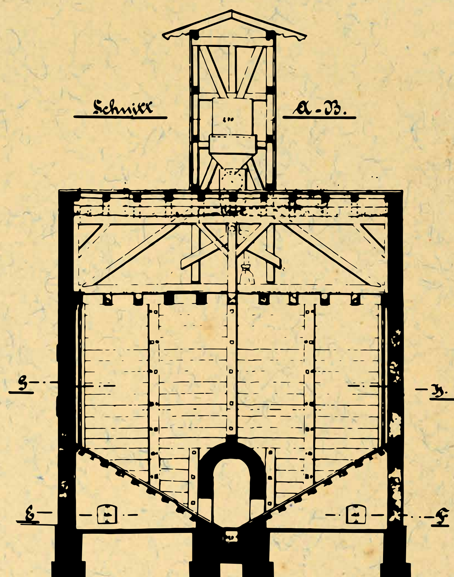
Przekrój zaprojektowanego magazynu zbożowego, 1889, APL sygn. 2590
